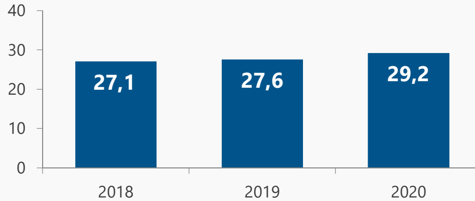
Consumo specifico forni - MJ/t clinker
