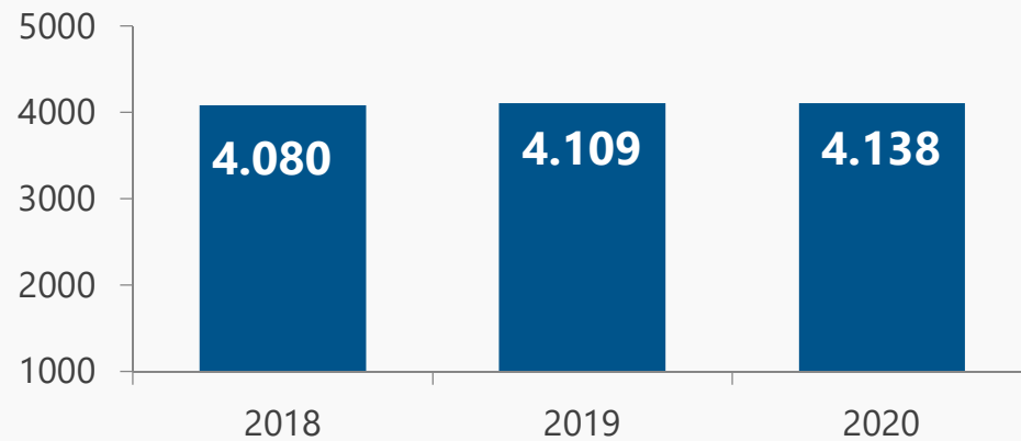
Consumo specifico forni - MJ/t clinker
