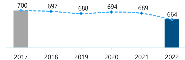
Emissioni dirette di CO 2 (lorde) - kg/t materiale cementizio
